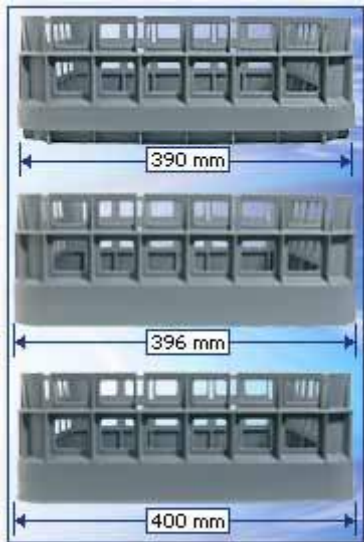
S 4x5/75 Trois dimension possible couvrant les standards machine 390 mm, 396 mm et 400 mm
